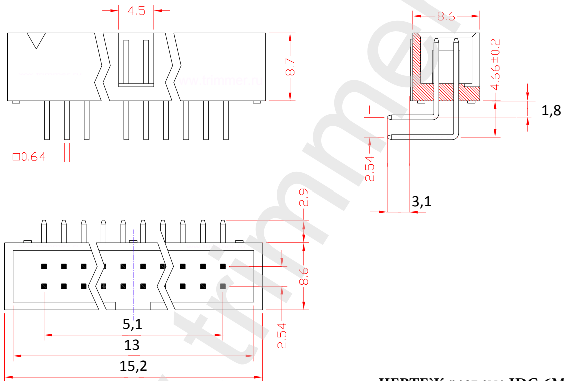
ЧЕРТЕЖ разъема IDC-6MR
