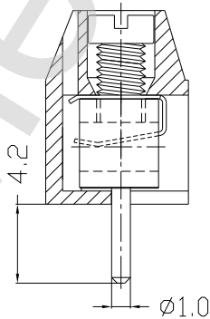
Клеммник на 2 контакта
