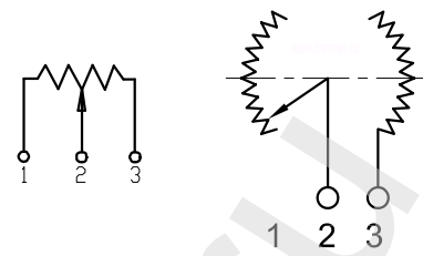
схема регулировки
