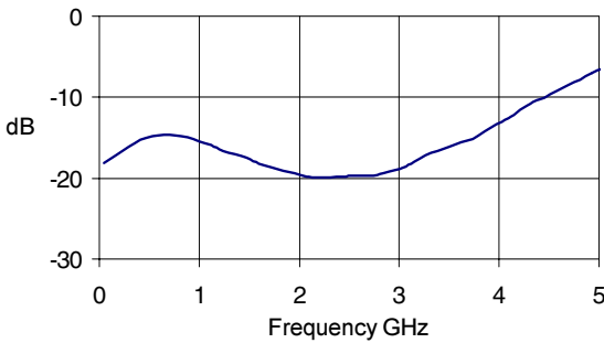
S11, I_D = 45\text{mA} , T = +25\text{C}
