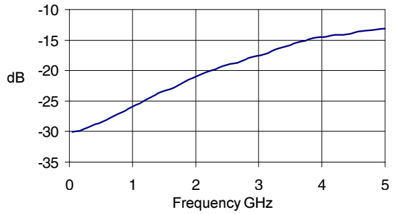
S12, I_D = 45\text{mA} , T = +25\text{C}
