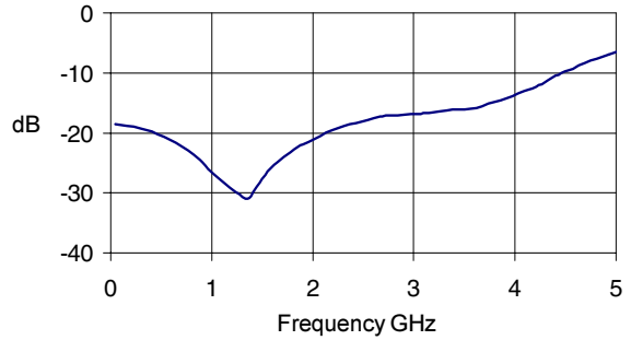
S22, I_D = 45\text{mA} , T = +25\text{C}
