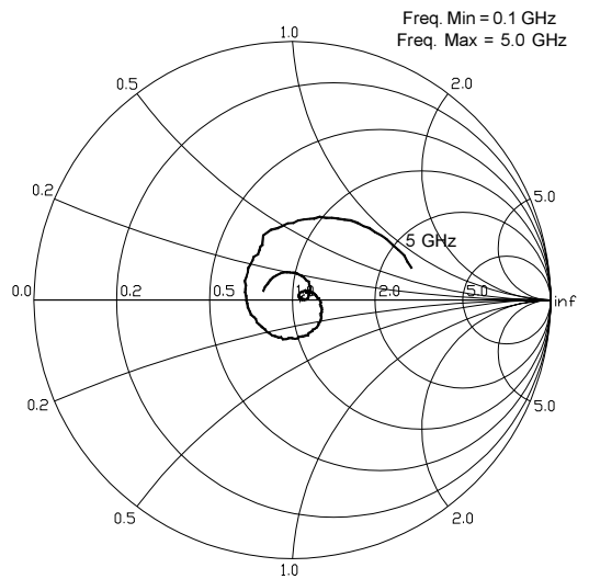
S22, I_D = 45\text{mA} , T_a = 25\text{C}
