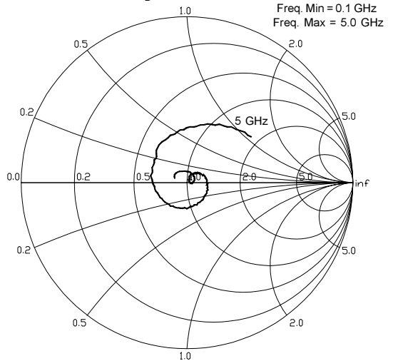
S22, I_D = 45\text{mA} , T_a = 85\text{C}
