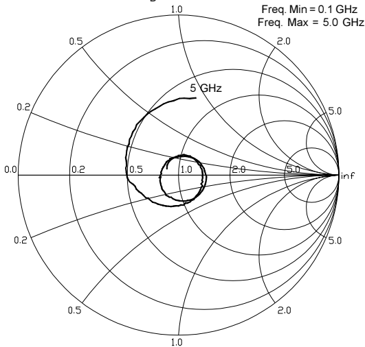
S11, I_D = 45\text{mA} , T_a = 85\text{C}
