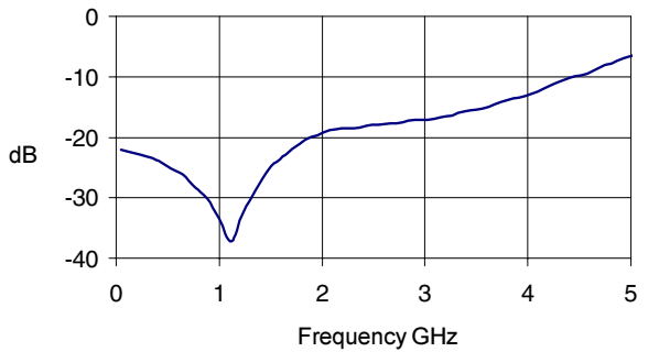
S22, I_D = 45\text{mA} , T = 85\text{C}
