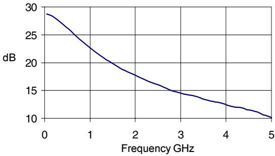
S21, I_D = 45\text{mA} , T = +25\text{C}
