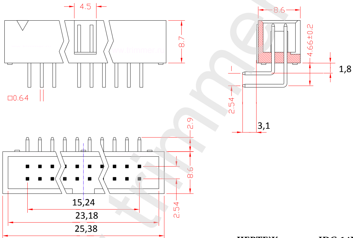
ЧЕРТЕЖ разъема IDC-14MR
