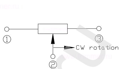
схема регулировки
