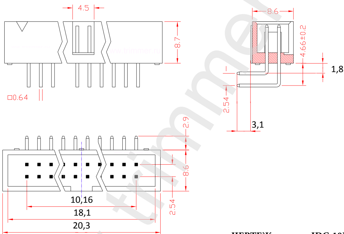
ЧЕРТЕЖ разъема IDC-10MR
